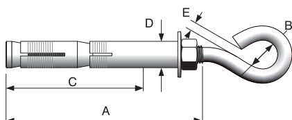
R2 – łącznik dwurozporowy
