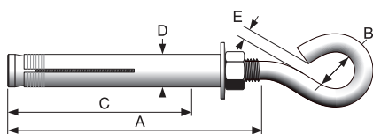
R1 – łącznik jednorozporowy
